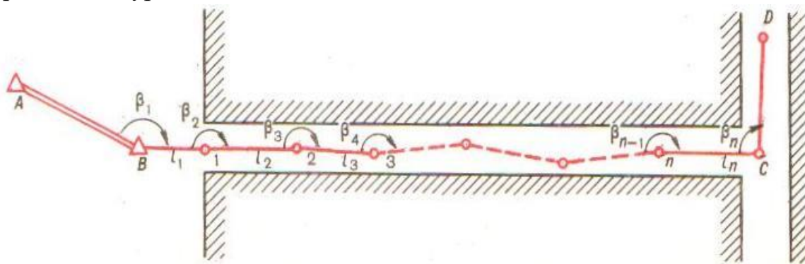
11-сурет. Штольня арқылы бағдарлаудың схемасы
