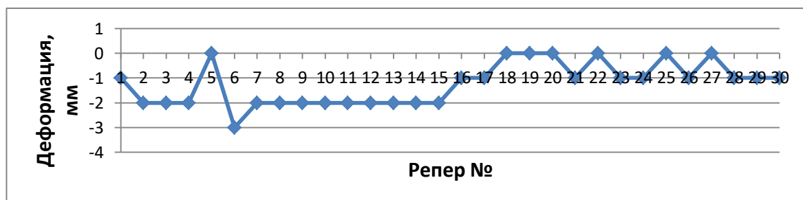
26-сурет. «Сарыарка» бекеті аймағындағы 2016-2019 жылдар аралығындағы реперлер деформациясының графигі
