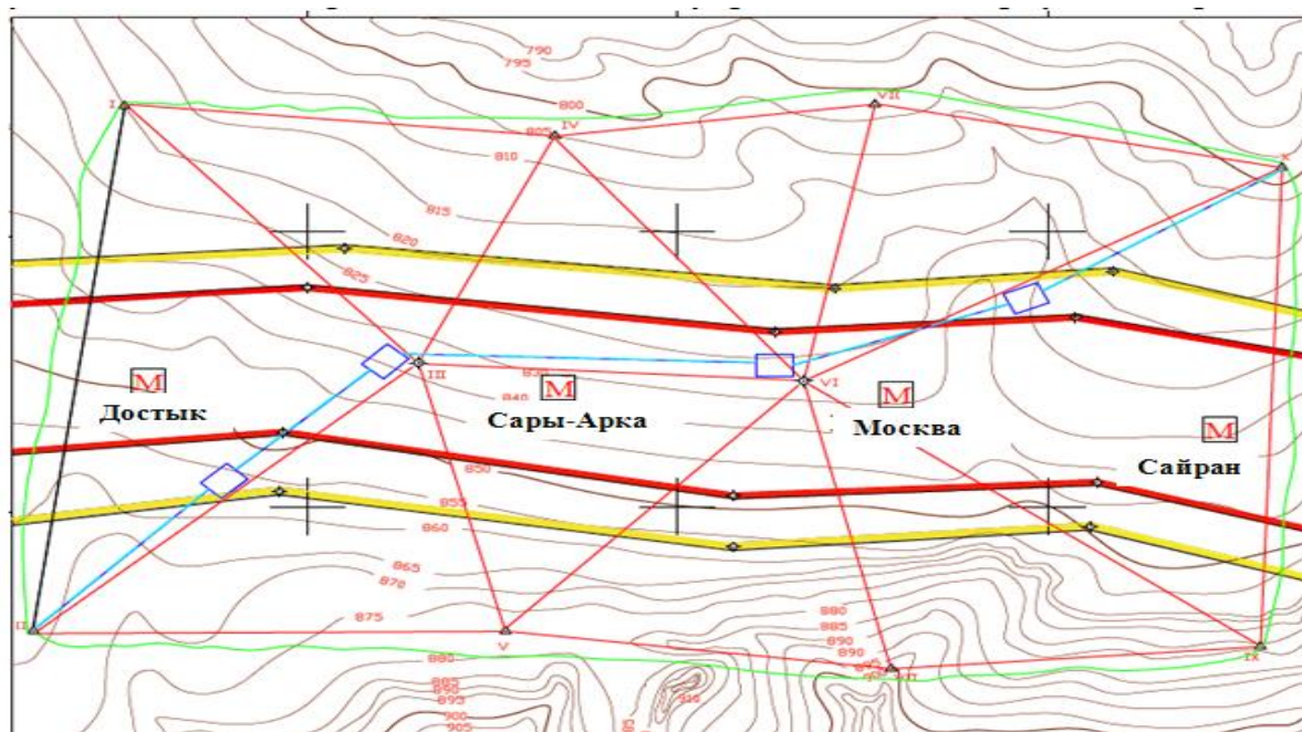
8-сурет. Геодезиялық тірек тораптары
