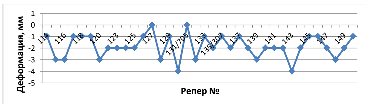
27-сурет. «Достық» бекеті аймағындағы 2016-2019 жылдар аралығындағы реперлер деформациясының графигі
